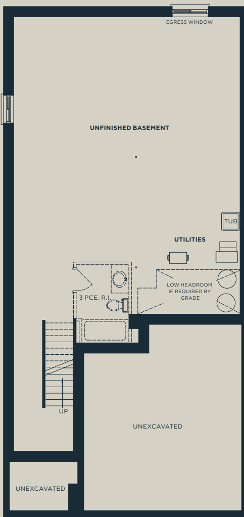
ELEVATION B
